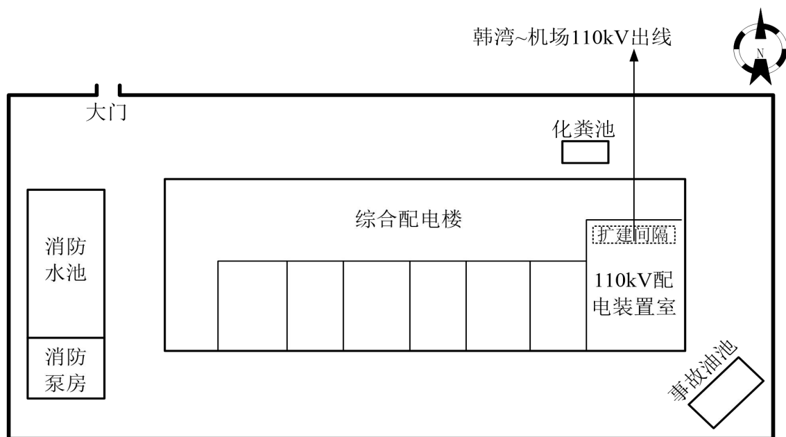
图 1-4 韩湾 110kV 变电站平面布置图
