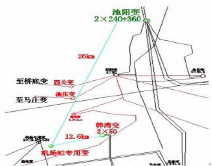
西咸国际机场三期供电工程地理接线图
