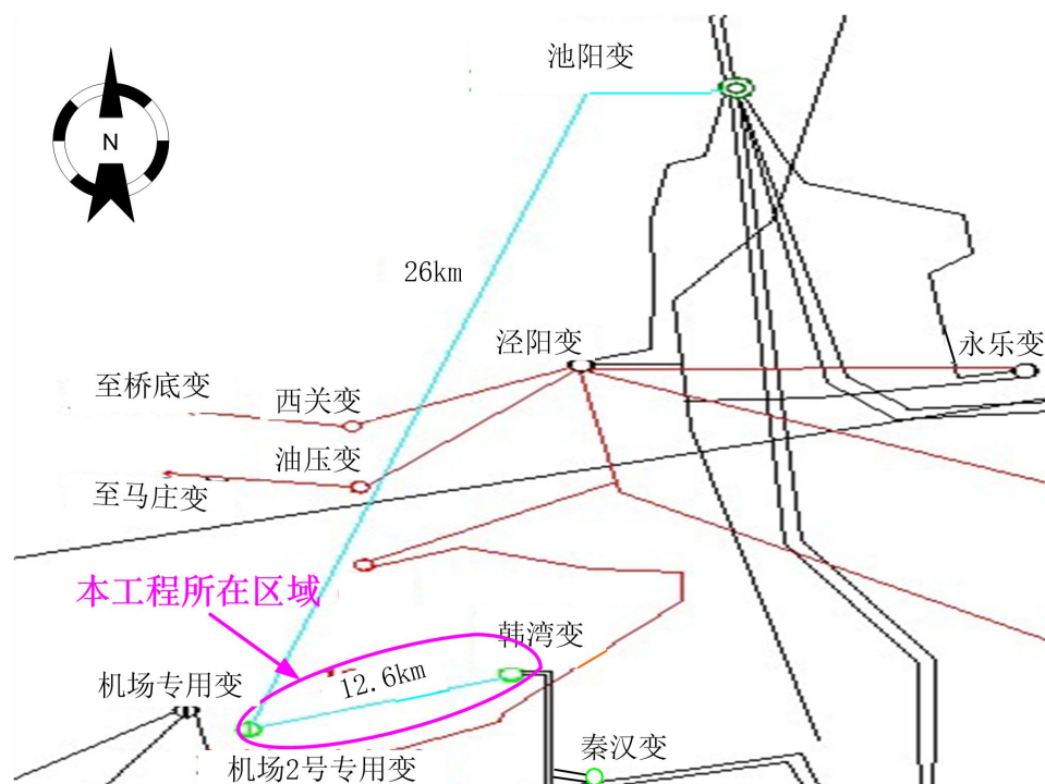
图 1-2 工程本期临时过渡接入方案示意图
