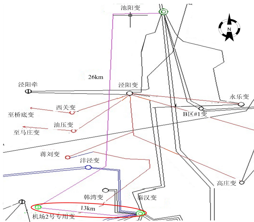
图 1-1 工程系统接入方案示意图
