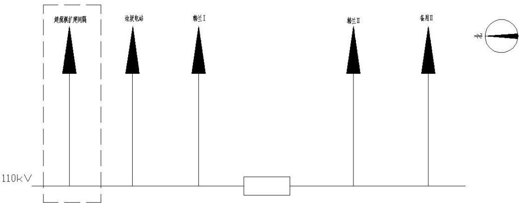
图 1-7 过渡期韩湾变 110kV 扩建间隔排列示意图
