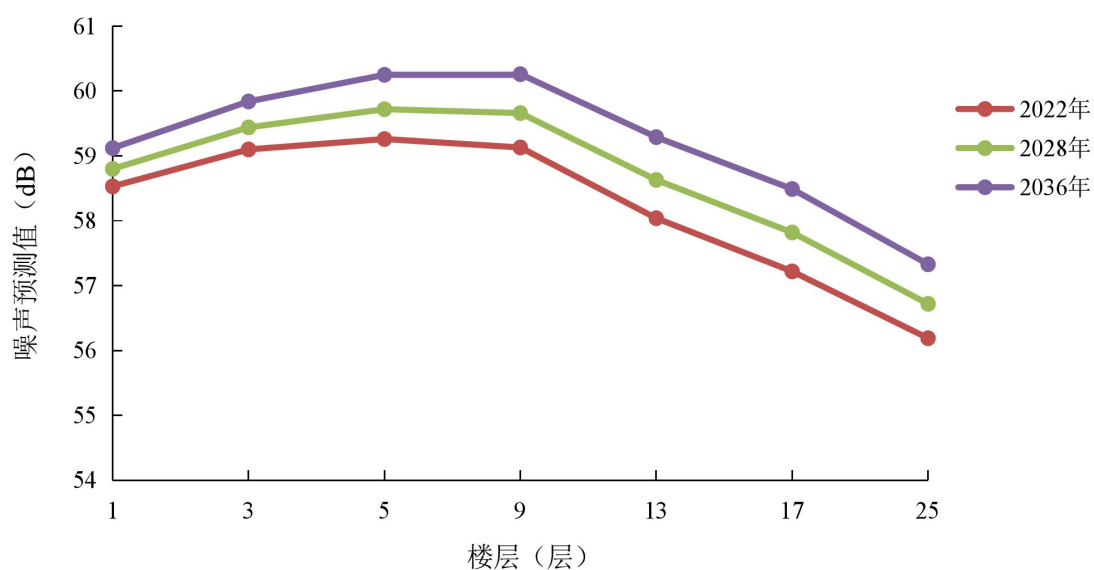
图 9-1 阳光城壹号上林悦 10 号楼各楼层噪声预测值垂向变化图（昼间）
