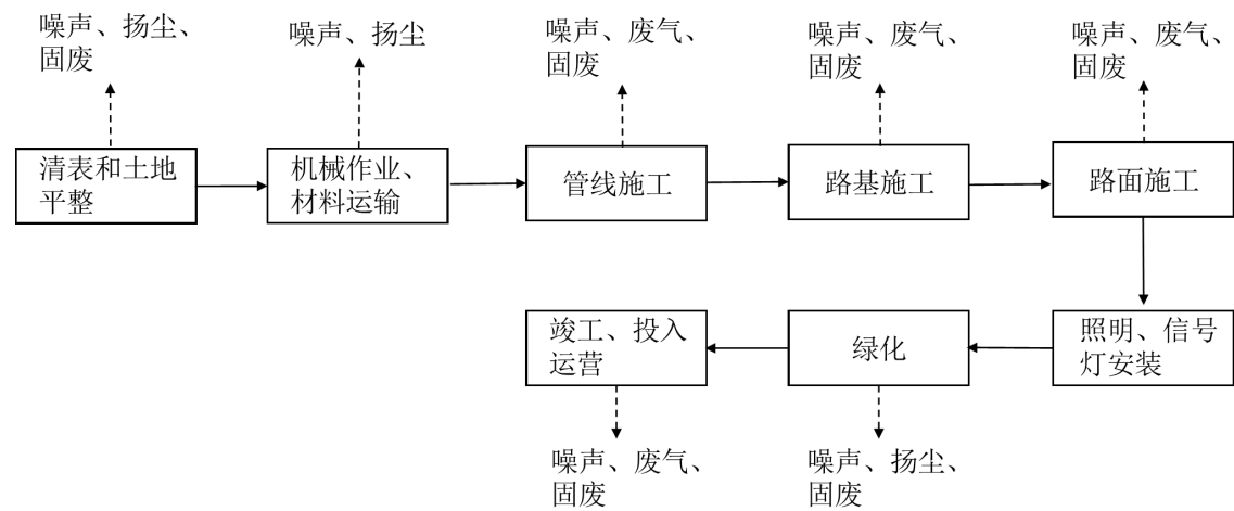
图 4 工艺流程及产污环节图
