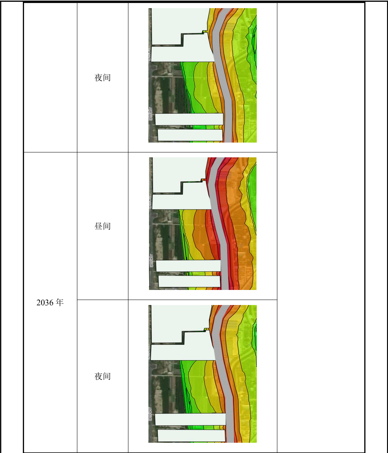
图 8 各特征年噪声等值线图
