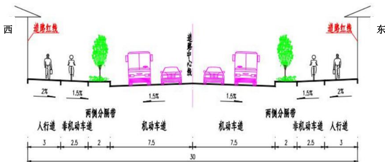
图 1 尚航六路（石化大道~丰裕路）标准横断面图
