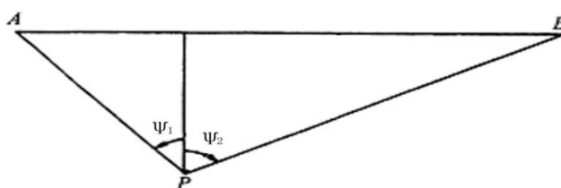
图 5 有限路段的修正函数示意图（A-B 为路段，P 为预测点）
