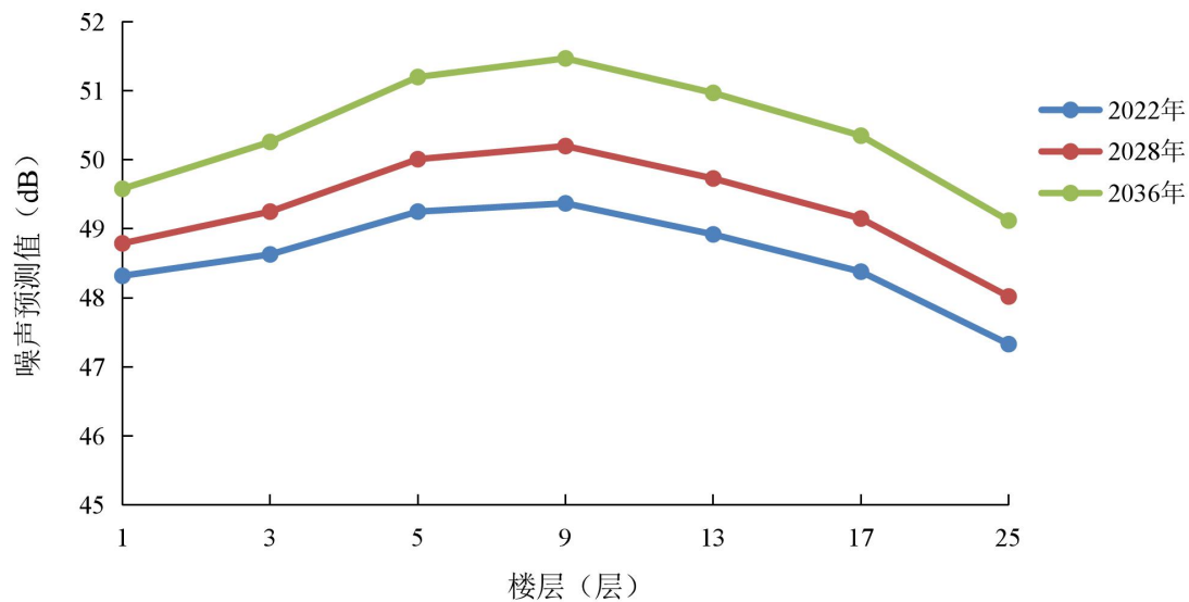
图 9-2 阳光城壹号上林悦 10 号楼各楼层噪声预测值垂向变化图（夜间）
