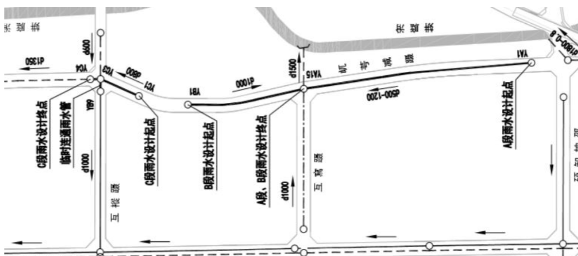
图 2 尚航六路（石化大道~丰裕路）雨水管道位置示意图
